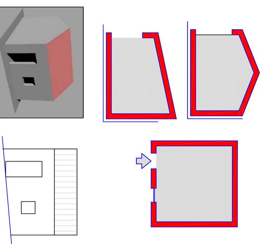
TIPO EDILIZIO N. 1 - MONOCELLULA A PIANO TERRA
