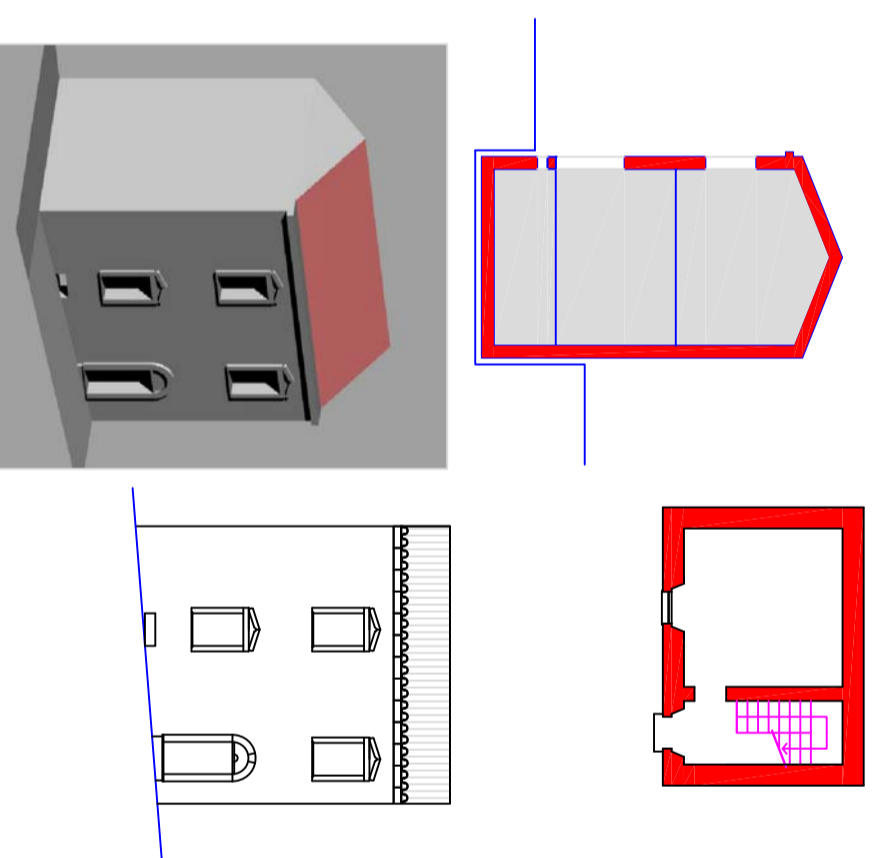
TIPO EDILIZIO N. 2 - MONOCELLULA SU DUE LIVELLI
