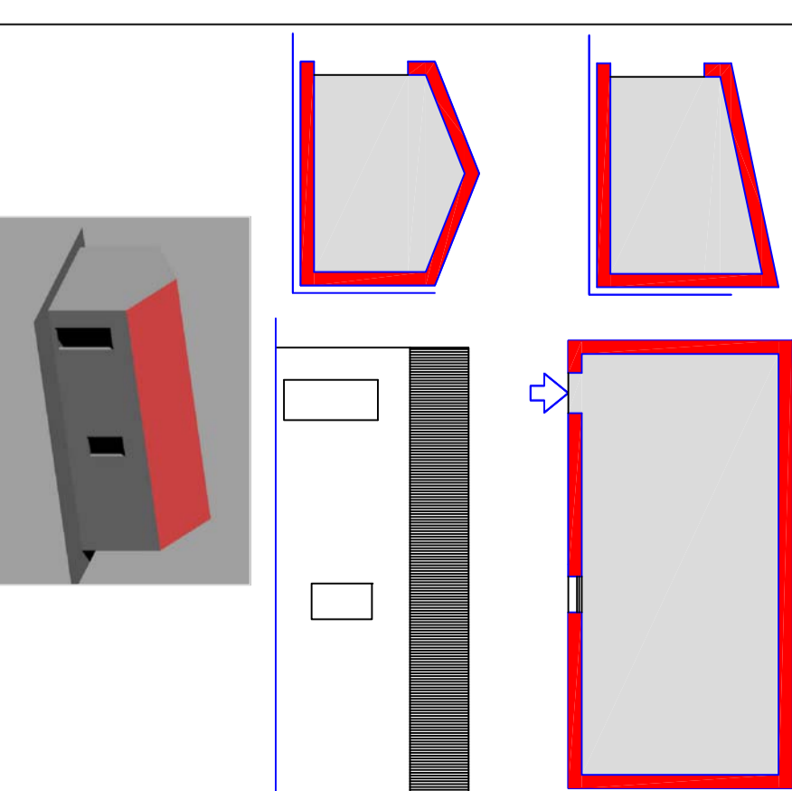
TIPO EDILIZIO N. 4 - DOPPIA CELLULA A PIANO TERRA
