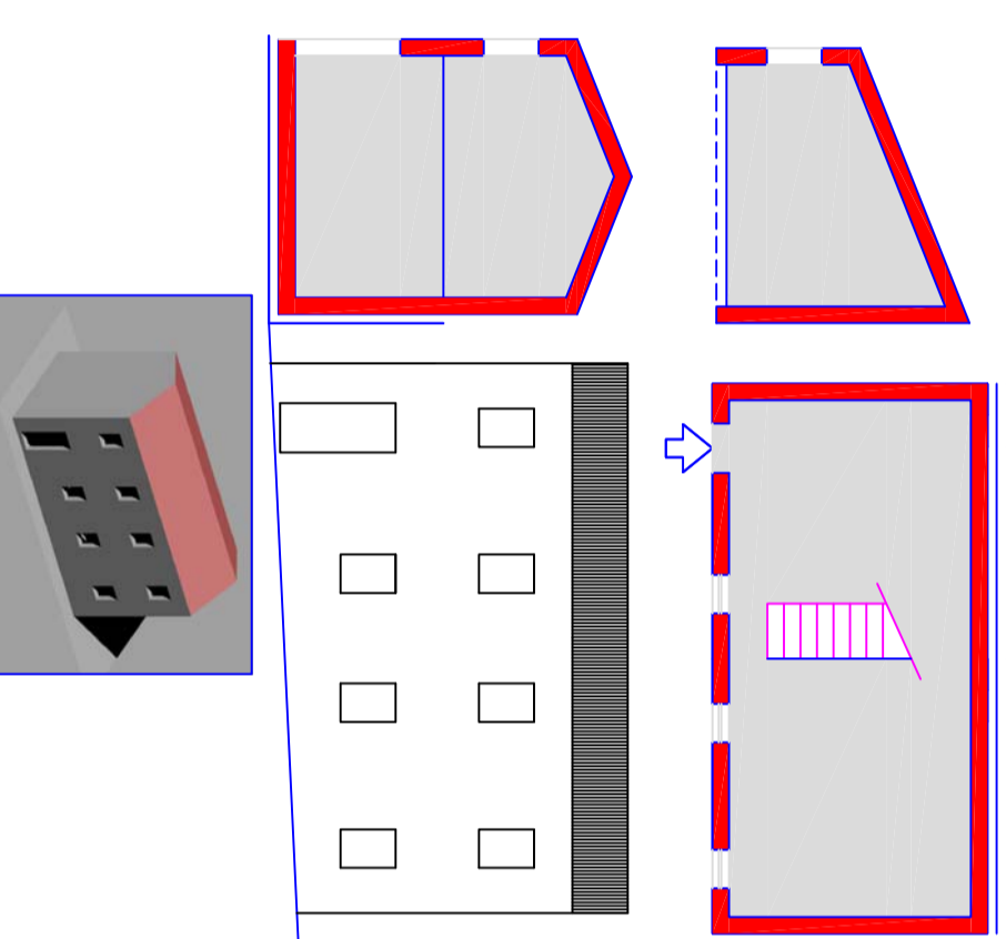
TIPO EDILIZIO N. 5 - DOPPIA CELLULA SU DUE LIVELLI
